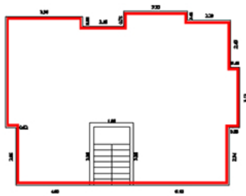
קומה 2
