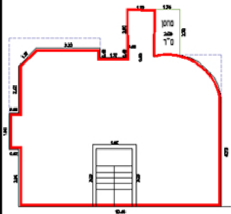
קומה 1
